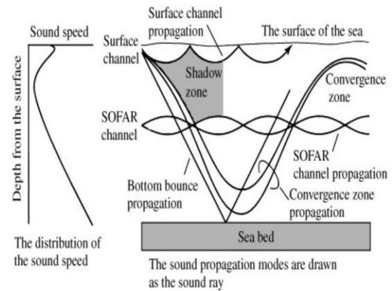
Gambar 6 Bentuk Propagasi Suara di Bawah Air (Kagawa et al., 2001)
